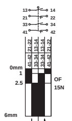
SPT 2NO/2NC Snap Action
